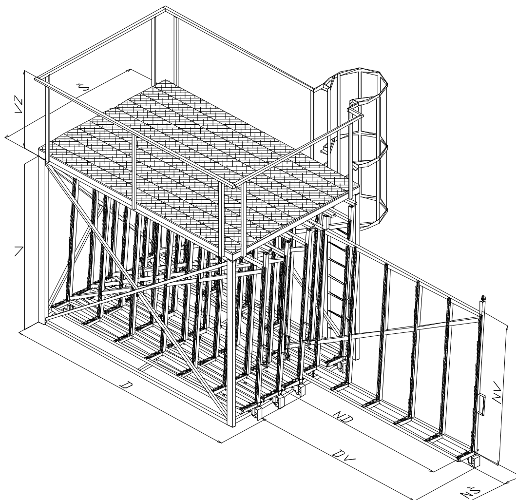
Obrázek – Typ ZH 04.5
